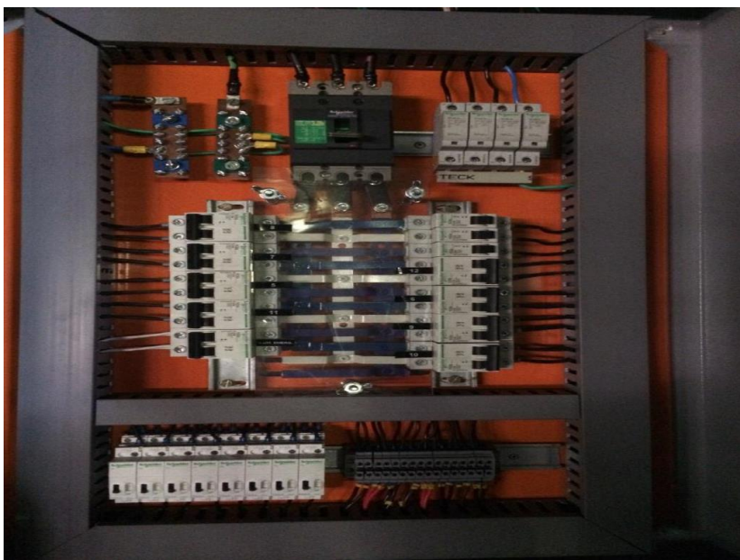
Imagem 26 – Quadro elétrico típico
